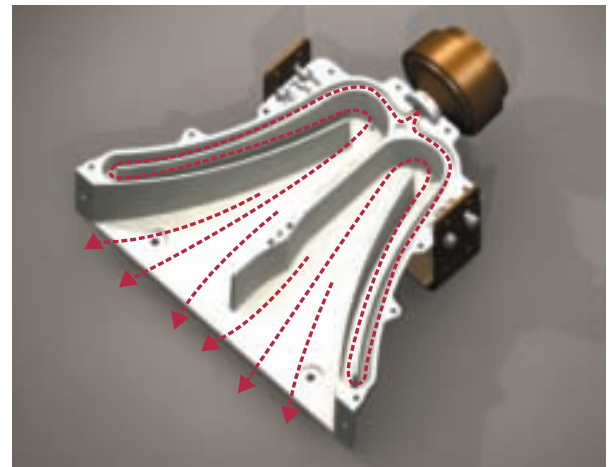
新開発の「レフレックスホーン」
