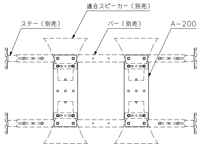
取付例（スピーカーを4本取り付けした場合） （縮尺：1/15）
