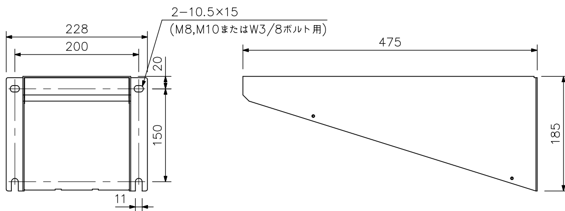
正面図
