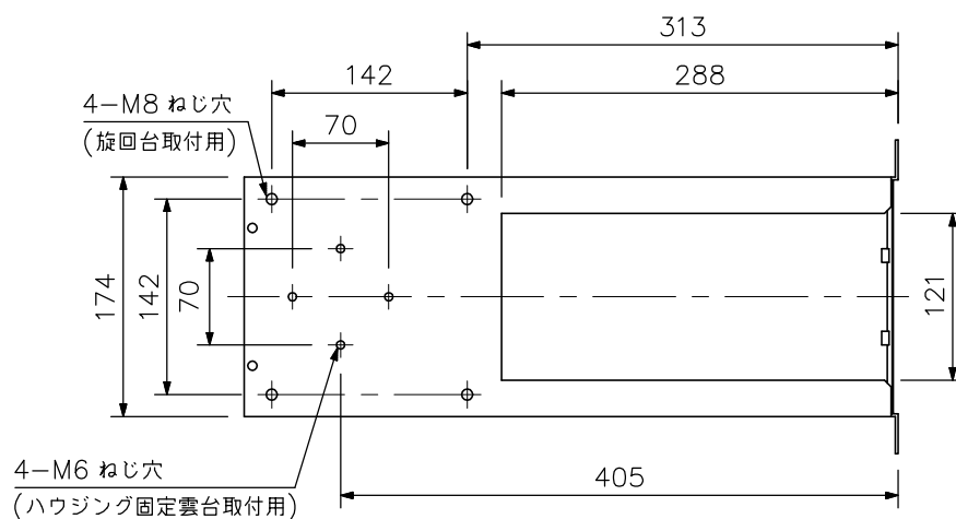
上面図
