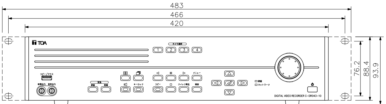
正面図
