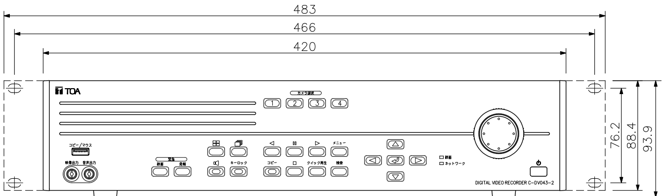
正面図
