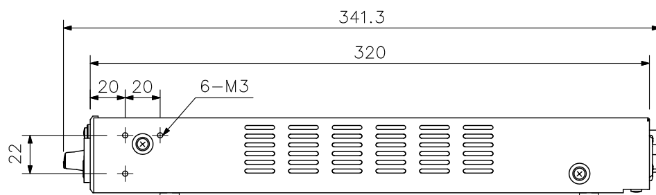
側面図
