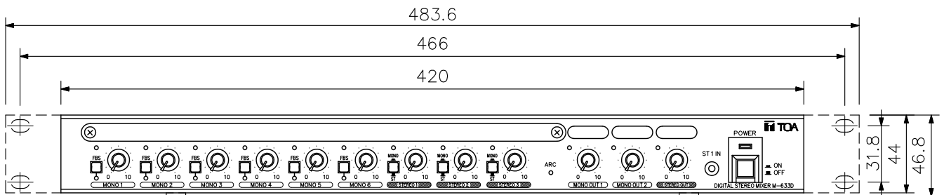
正面図
