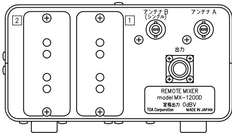
背面図
