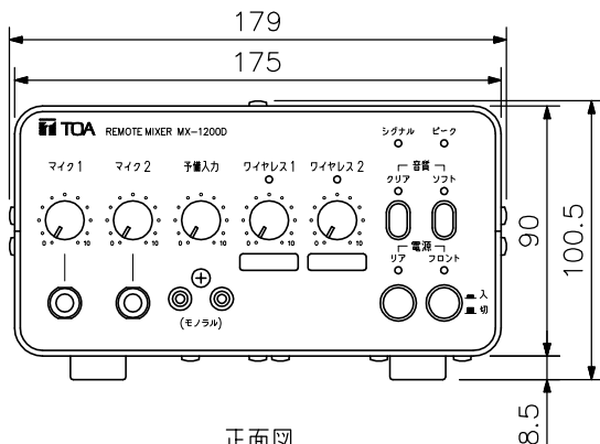
正面図
