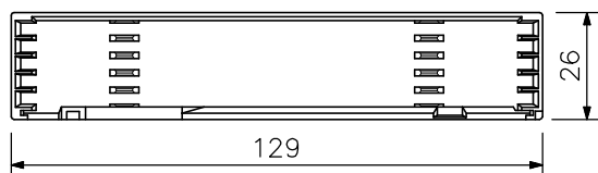
正面図
