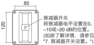
[前端]
