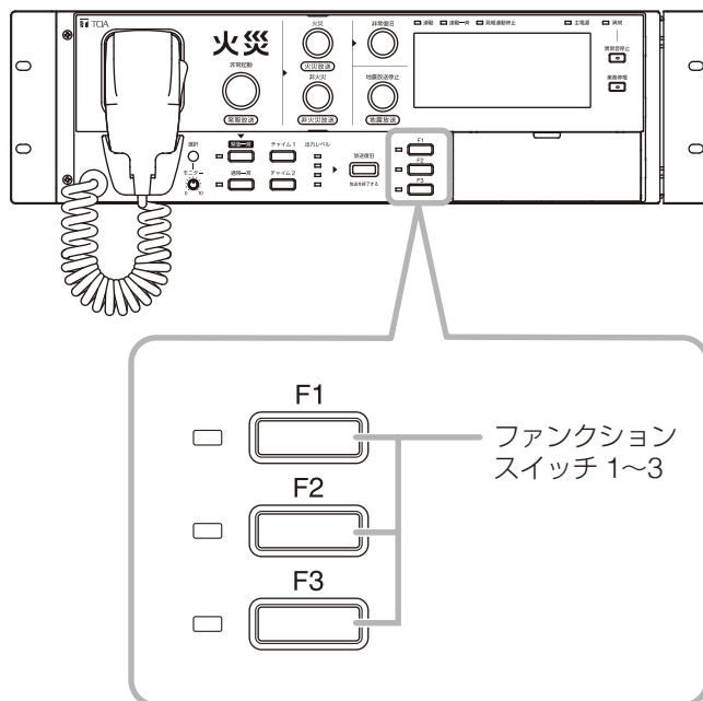
FS-A2500EP (操作部)
