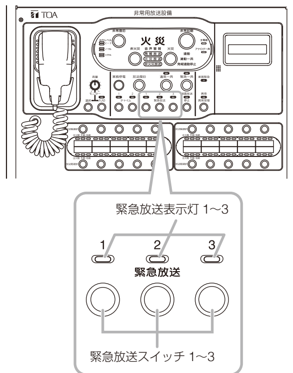
FS-1010RM/1020RM/1030RM 操作部
