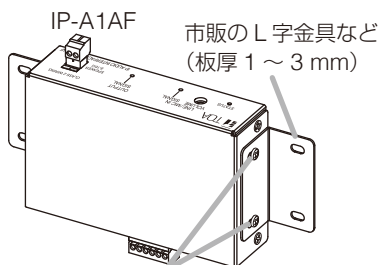
小ねじ M3×6 (付属品、左右 4 カ所)
