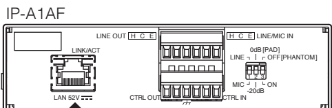
PoE+ または PoE スイッチングハブから
