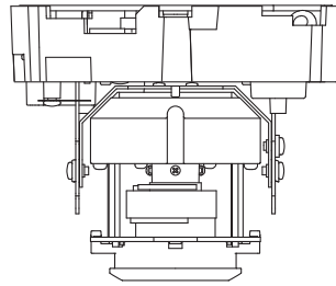
[ドームカバーを外した正面図]
