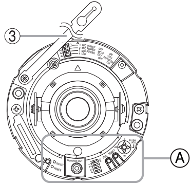
[ドームカバーを外した底面図]
