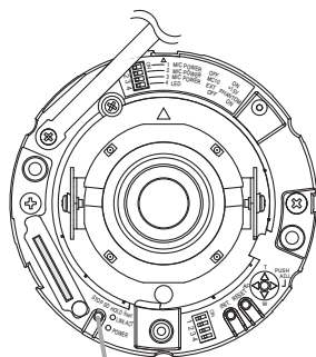
SD録画停止スイッチ
