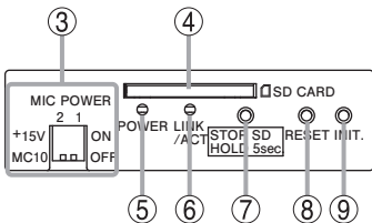
[背面端子部 拡大図]
