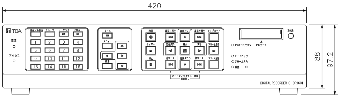
正面図
