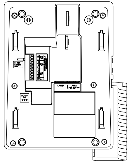
底面図
