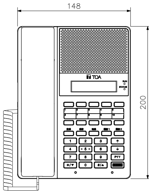
上面図
