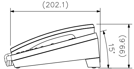
スタンド取付図(縮尺:1/5)
