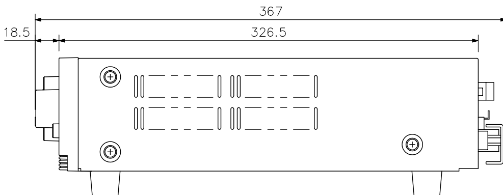
側面図
