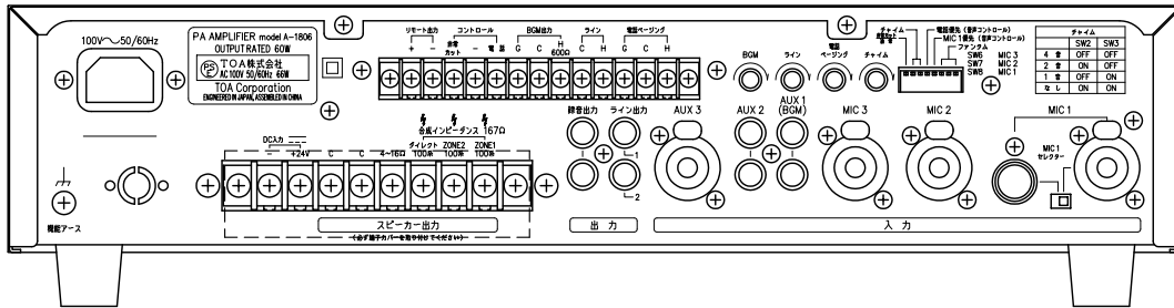
背面図
