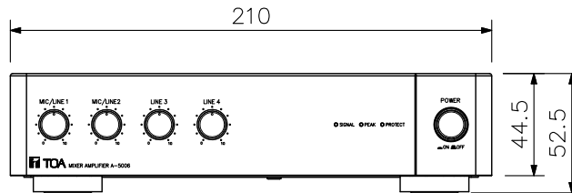
正面図
