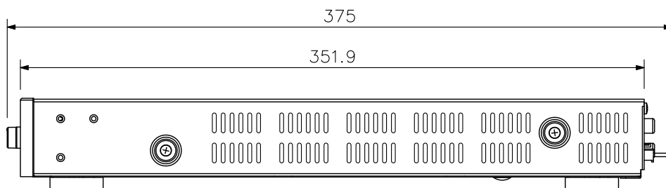
側面図
