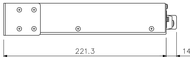
側面図
