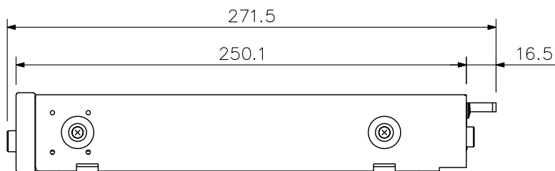
側面図
