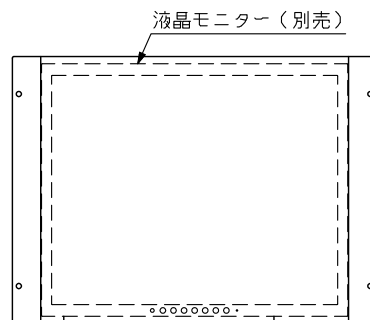
取付例 (縮尺: 1/10)
