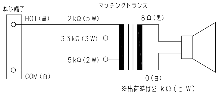
結線図
