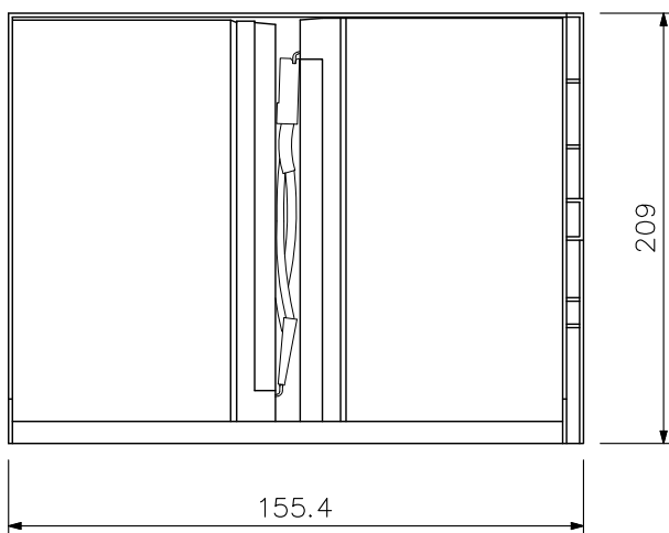
側面図
