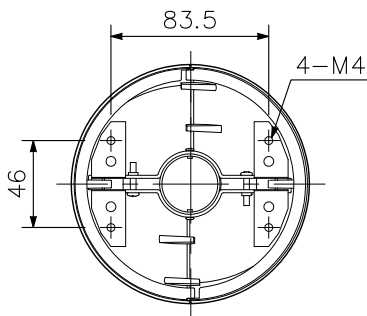
カメラ取付金具用穴寸法
