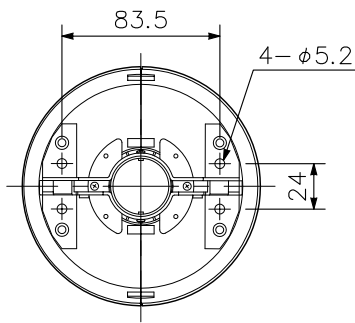
二重天井取付用穴寸法
