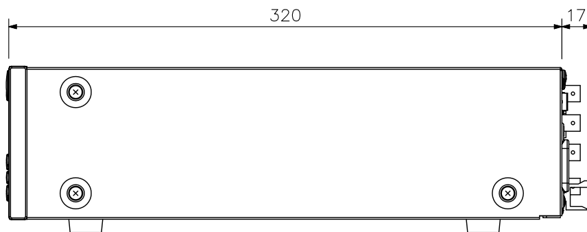
側面図
