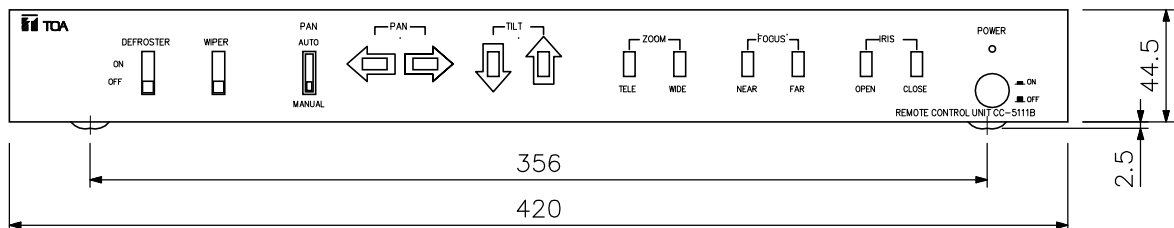
正面図
