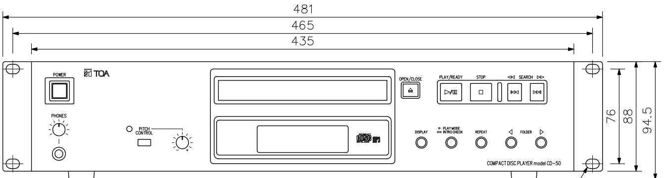
正面図
