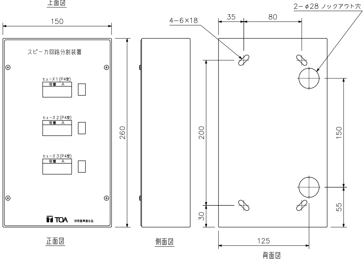
上面図
