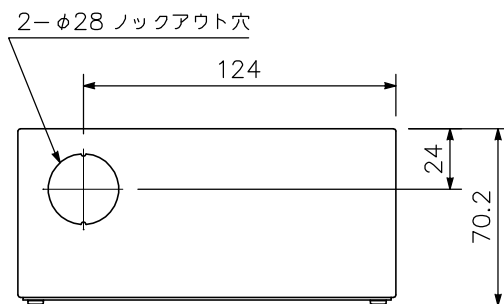
上面図
