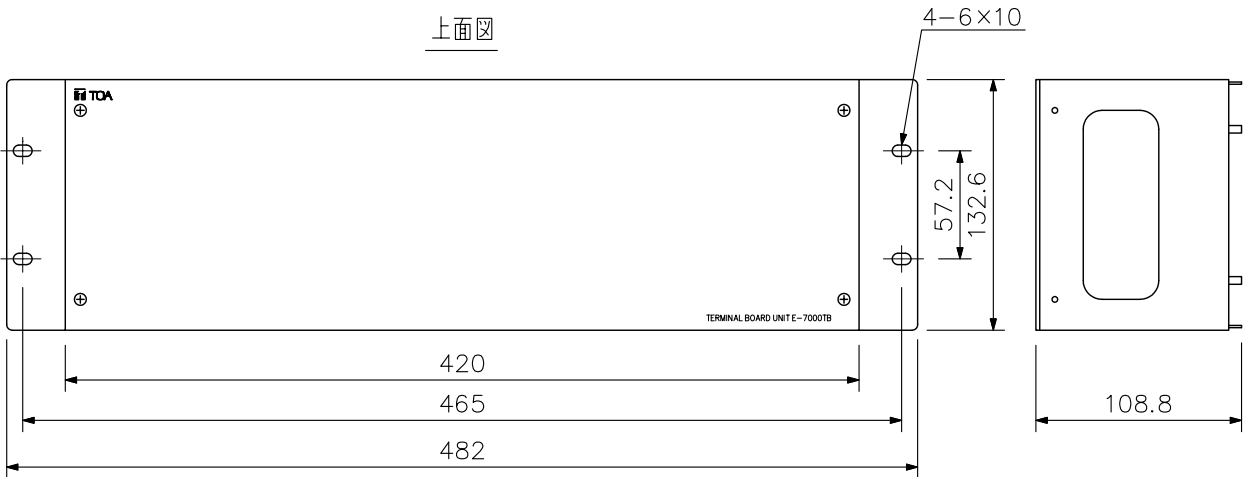
正面図
