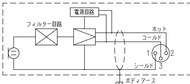
回路図
