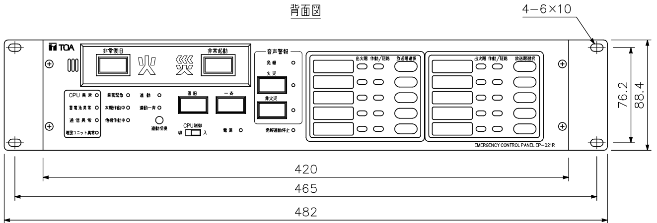
正面図
