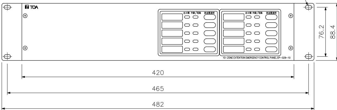
正面図
