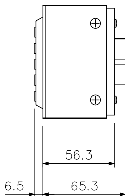
側面図
