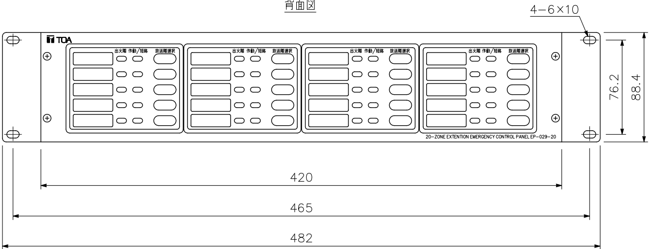
正面図
