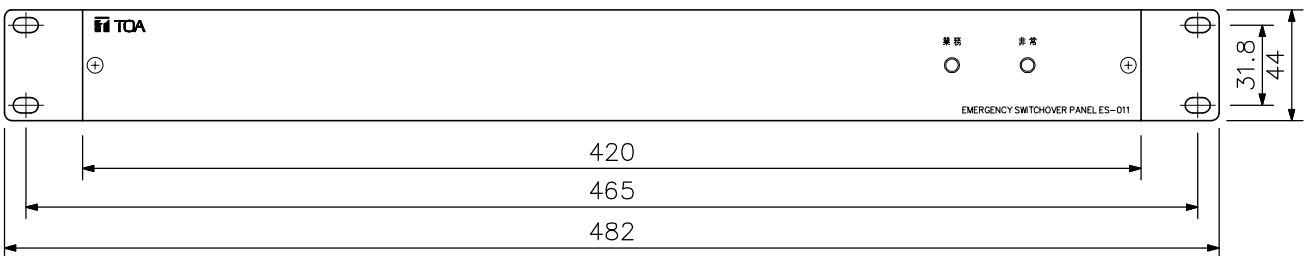
正面図
