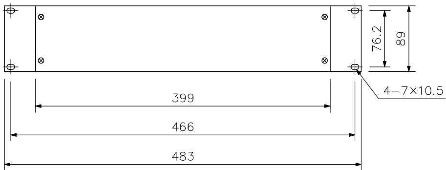
正面図
