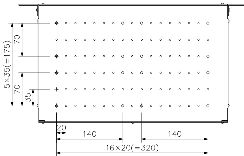
底面図
