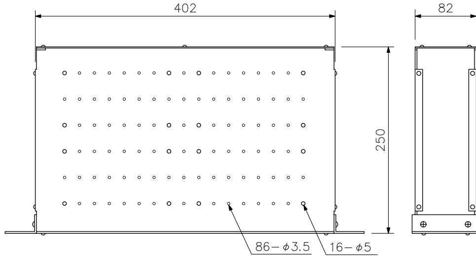
上面図
