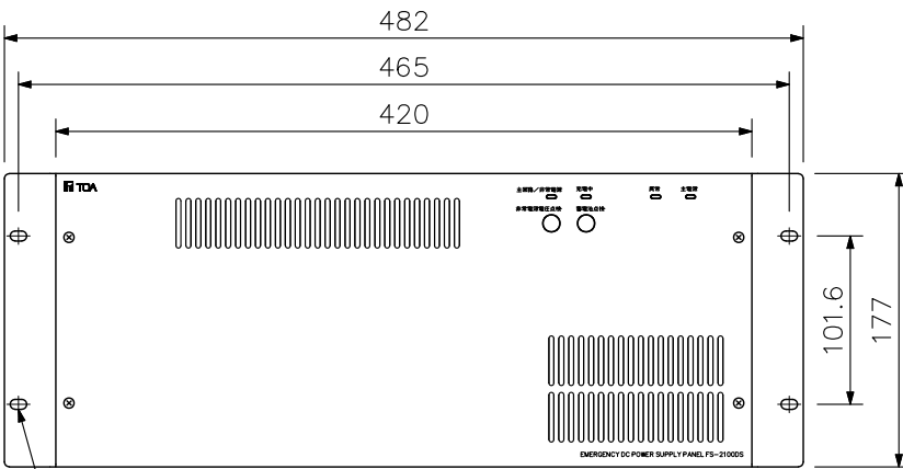
正面図
