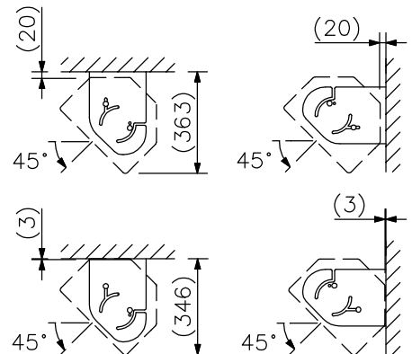
ES-0851を壁や天井に密着させて取付けた場合の振り角度
