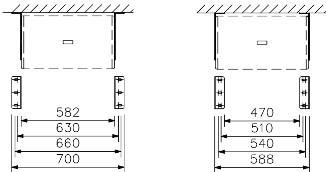
金具が外向きになるようにES-0851を取り付けた場合の取付寸法
