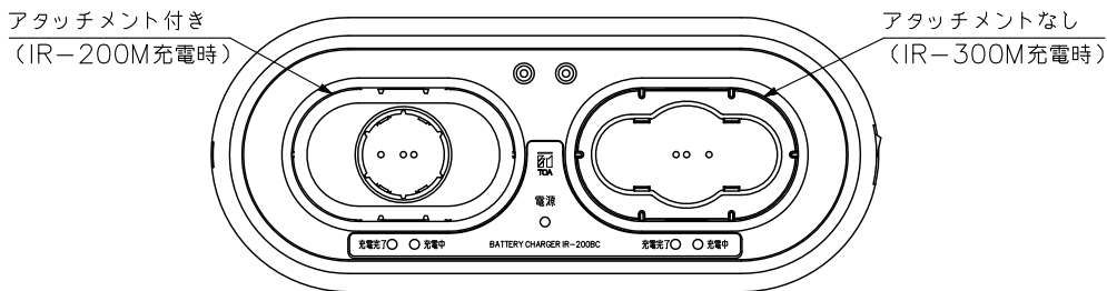
上面図
