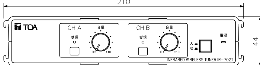
正面図
