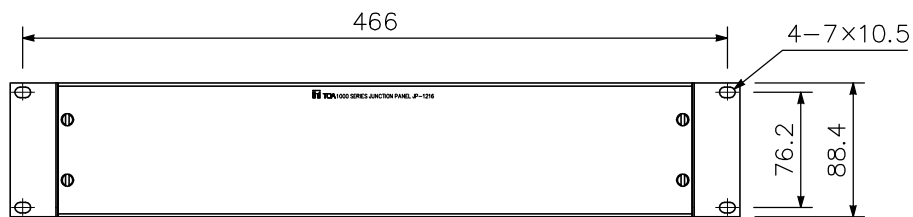
正面図
