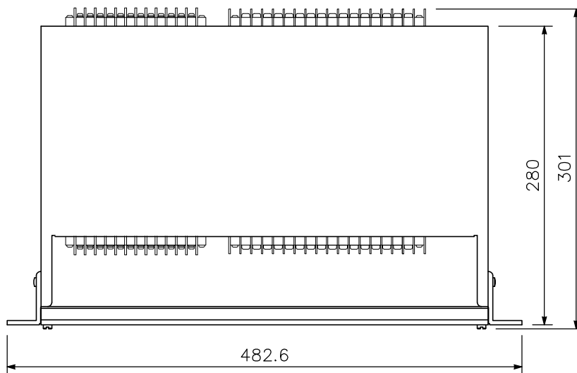
上面図
