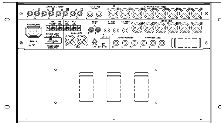
背面図
