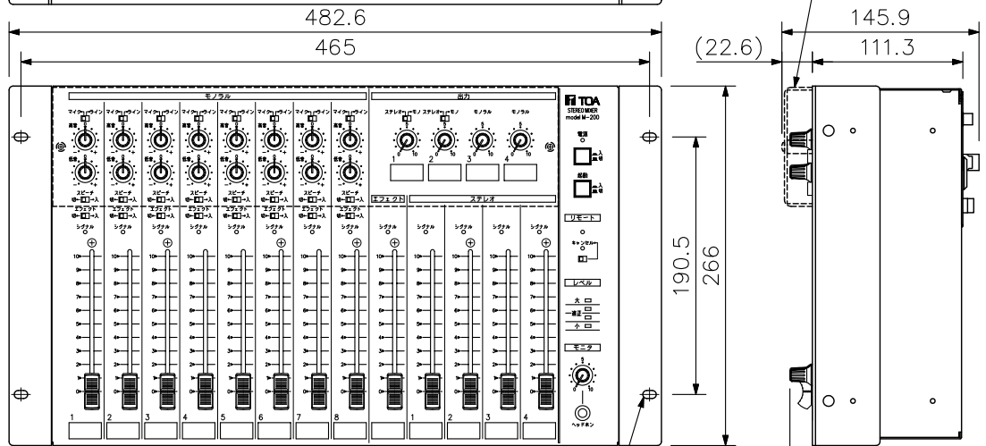
側面図
