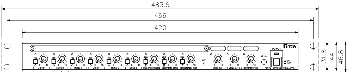
正面図
