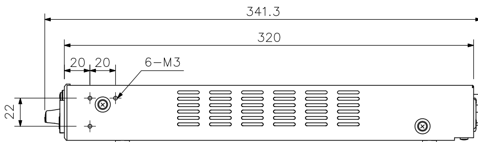
側面図
