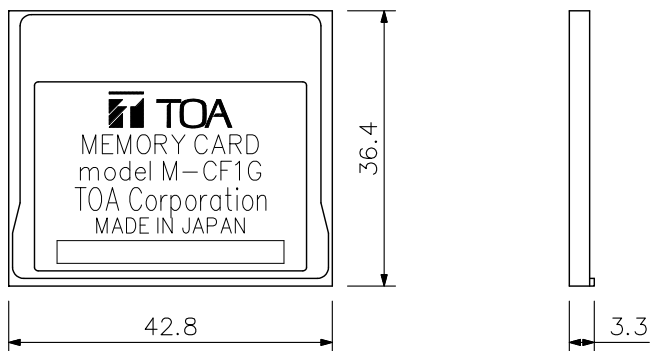
正面図
