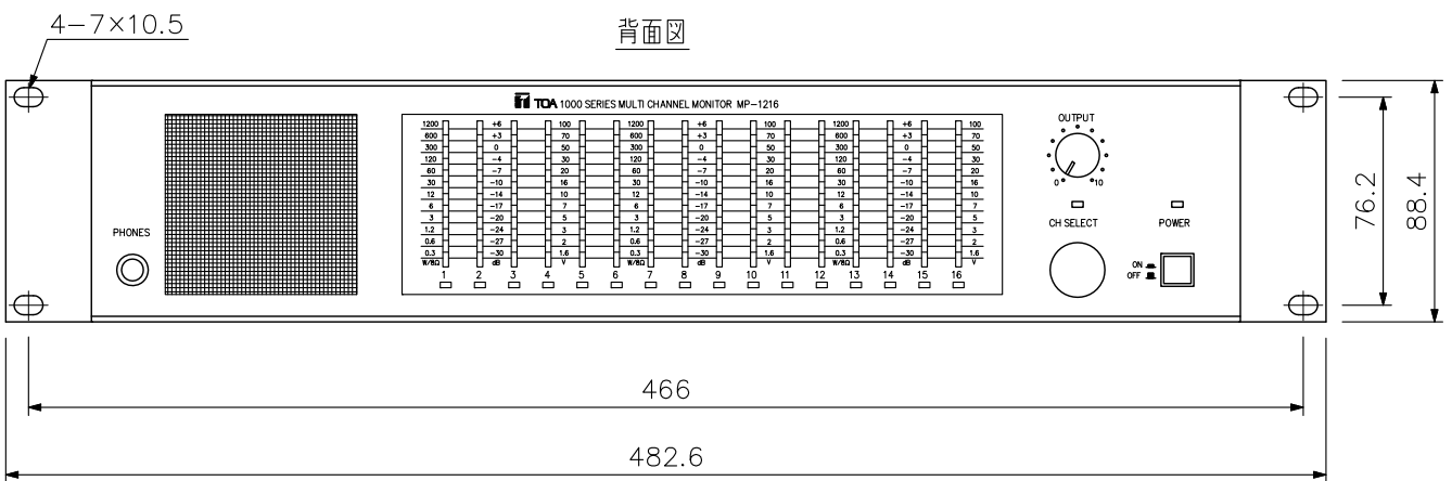
正面図
