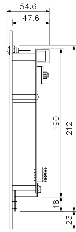
側面図
