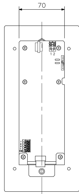
背面図
