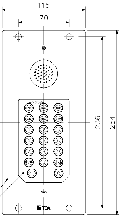
正面図
