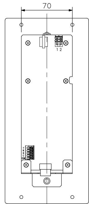
背面図
