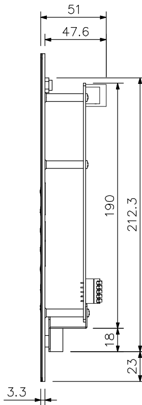
側面図
