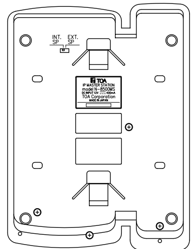
据置図（縮尺：1/5）
