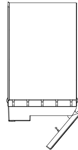
フロントカバーを開いた上面図 （縮尺：1/3）
