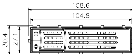
正面図
