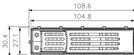
正面図
