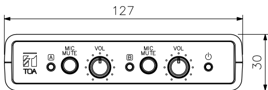
正面図
